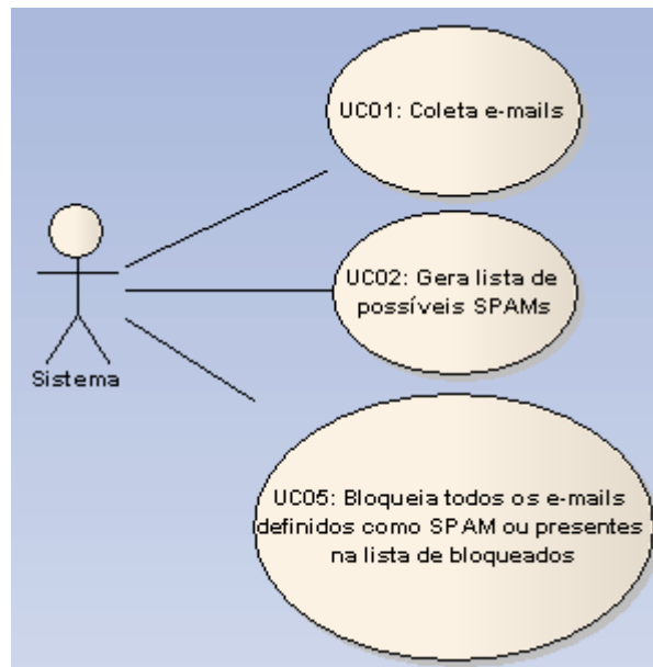
Figura 01: Diagrama de caso de uso da ferramenta.
