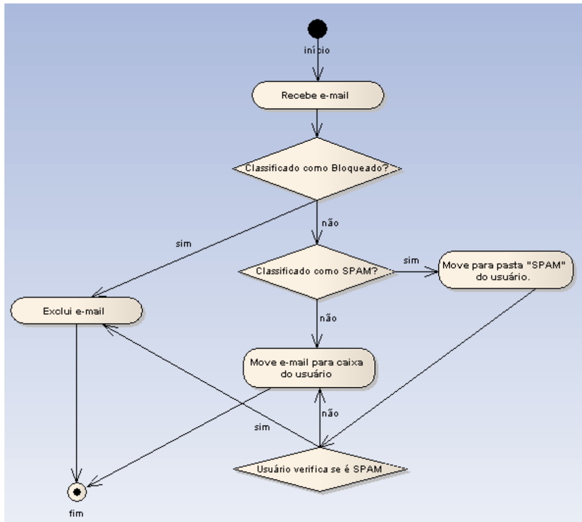
Figura 03: Diagrama de atividades.
