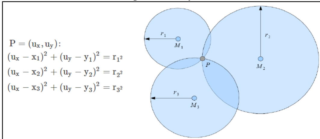
Figura 3 - Trilateração
