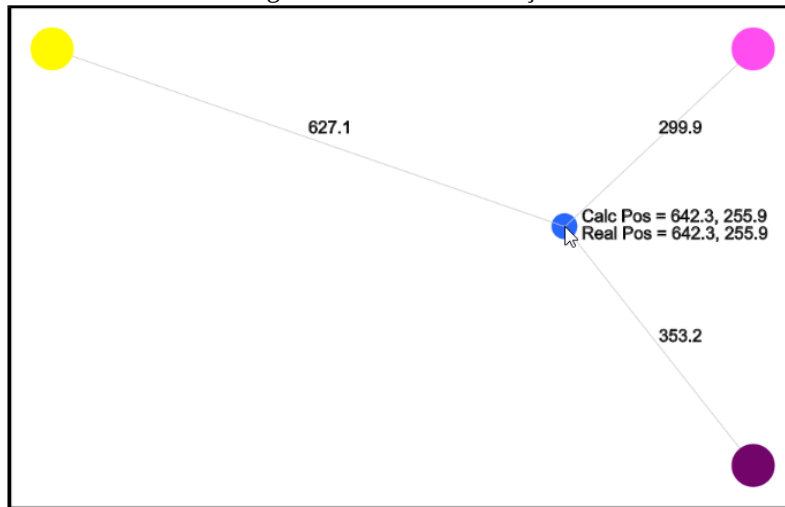
Figura 11 - Testes trilateração
