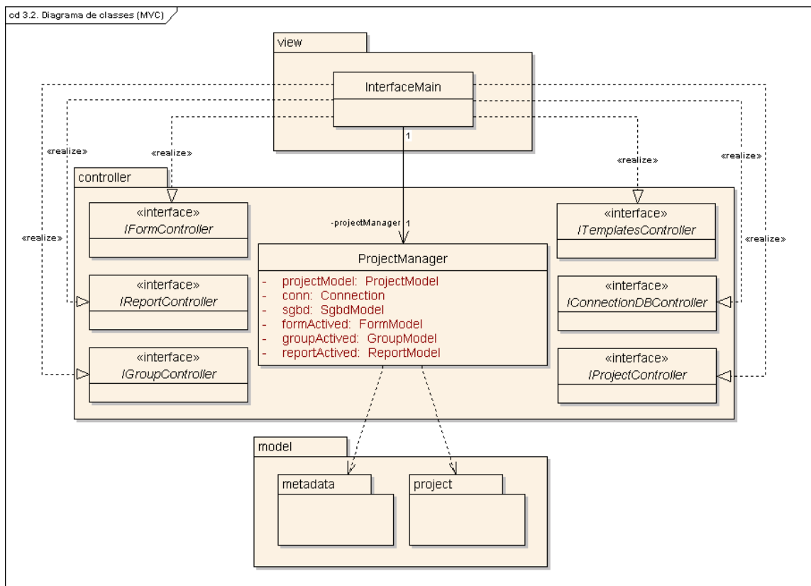
Figura 8 – Diagrama de pacotes descrevendo o padrão MVC aplicado na ferramenta
