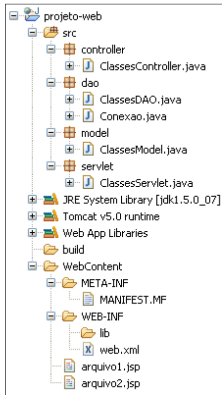
Figura 42 – Copiando arquivos gerados para o projeto web
